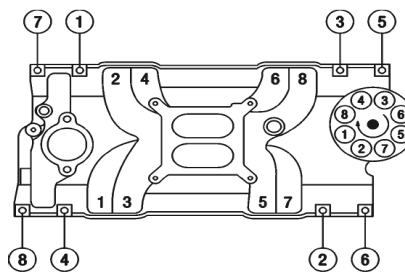
ORDRE D'ALLUMAGE 1-8-4-3-6-5-7-2
