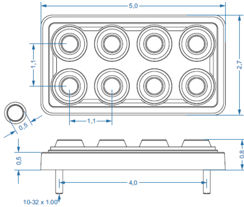
SwitchPanel-8 Mini
